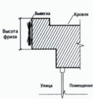
Высота подложки меньше высоты фриза
