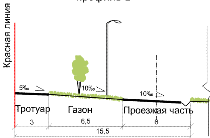
ул. Большая Балашиха профиль Б
