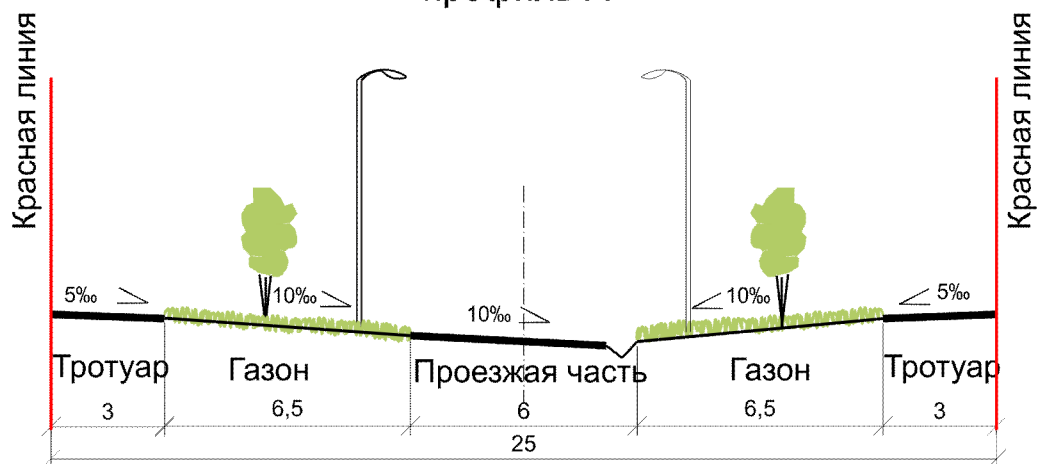
ул. Большая Балашиха профиль А
