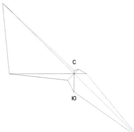
Рисунок 3.1 – Роза – диаграмма ветров
